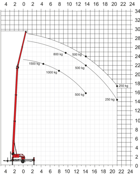
Lastdiagramm Hakenbetrieb
